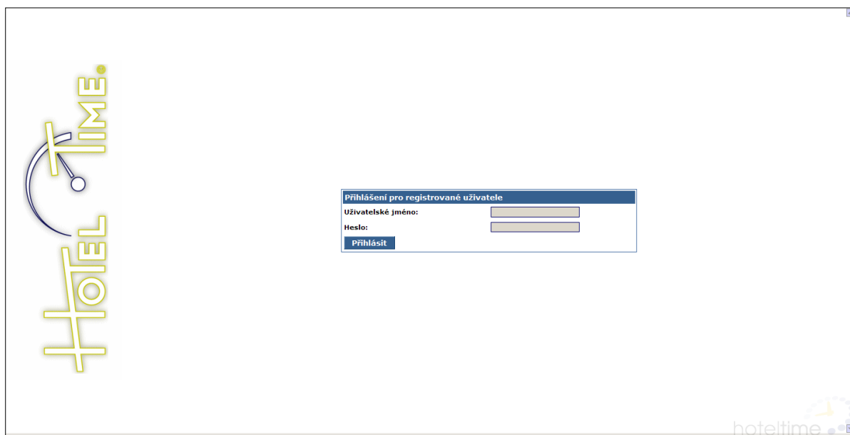
Obrázek 2 - přihlášení
