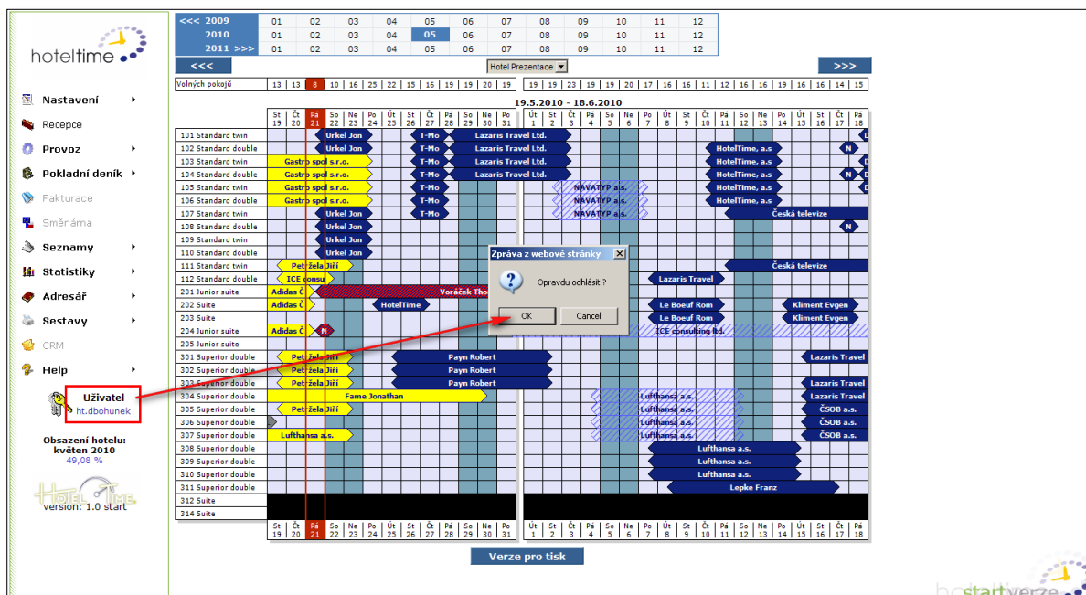
Obrázek 3 - odhlášení
